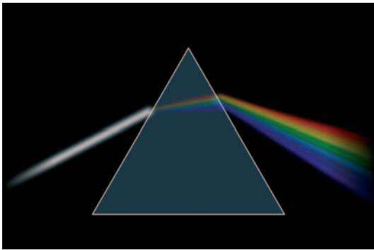
2- Décomposition de la lumière blanche dans un prisme
