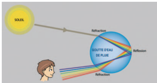
3- Passage de la lumière blanche dans une goutte d'eau
